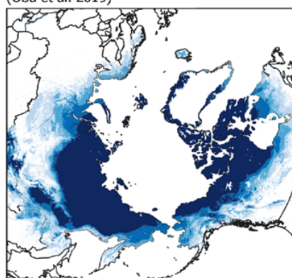
d) GlobPermafrost, 2000-2016 (Obu et al. 2019)
